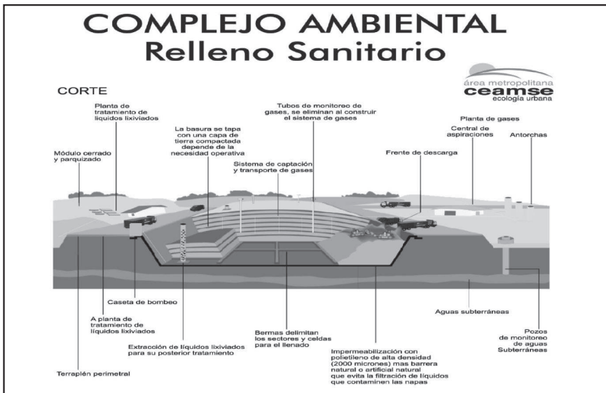
Figura 9.4. Relleno sanitario
