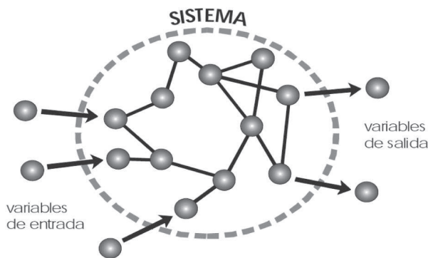
Figura 11.3. Sistema abierto
