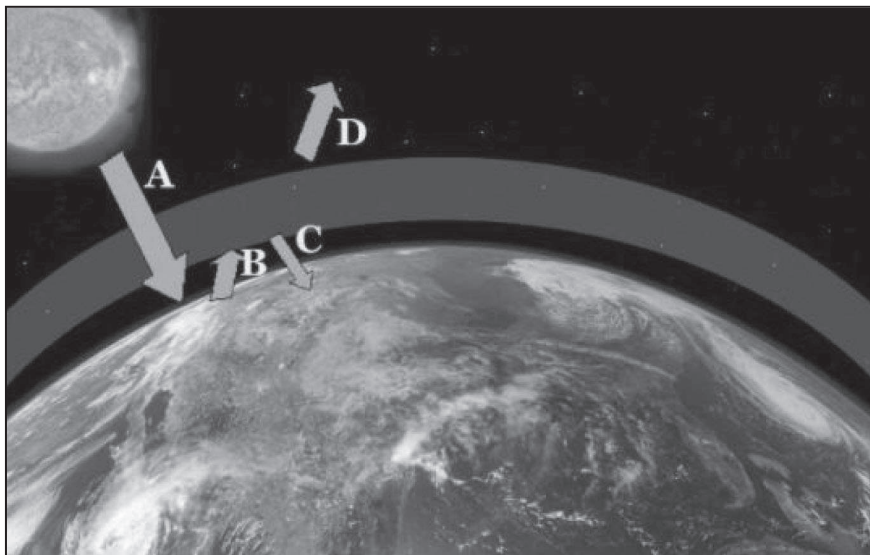
Figura 9.8. Efecto invernadero
