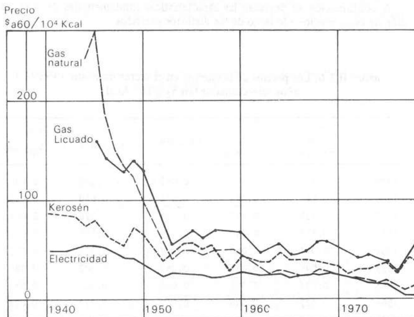
Gráfica II.1.2 Los precios reales de la energía en el sector doméstico 1939-1977
