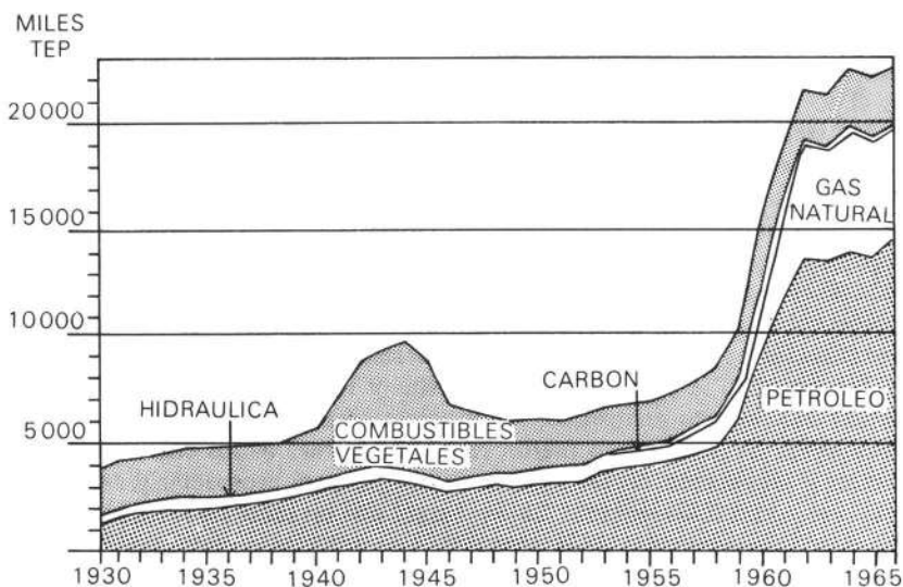
Gráfica I.2.1 La producción de energía primaria por formas 1950-1965
