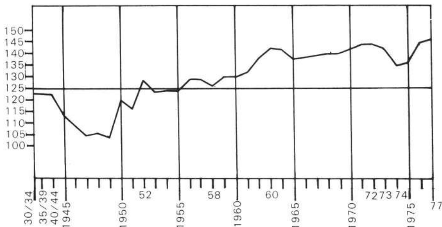
Gráfica I.3.4 Evolución del contenido energético del producto interior bruto de Argentina 1930-1977 (Kep/U$ 1965)
