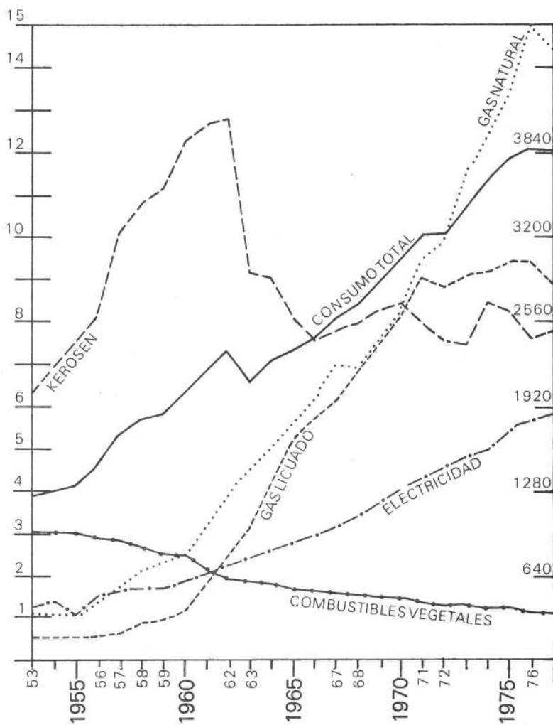
Gráfica II.1.1 El consumo de energía por formas en el sector doméstico ( 10^3 TEP)
