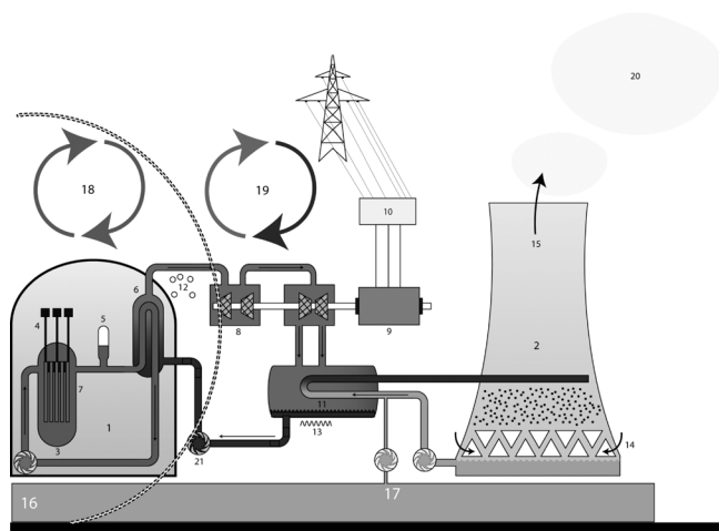
Figura 5: Esquema de un reactor nuclear (tipo PWR).
