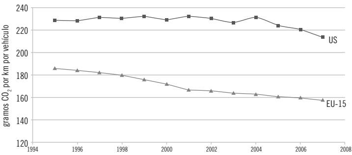
Figura 4: Emisión de CO2 por vehículos livianos, EU-15 y US. Fuente: EU Commission, US Department of Transport.
