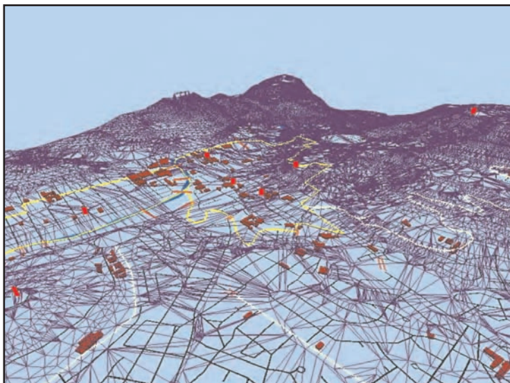
MDT aspecto de hilos de triangulación TIN
