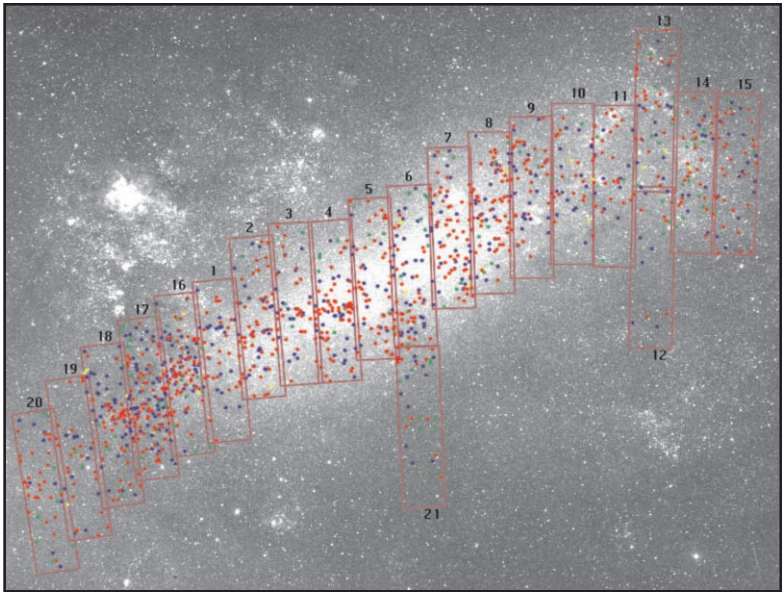
El gráfico de las estrellas de la Nube Mayor de Magallanes fue elaborado con el Software origin 8.
