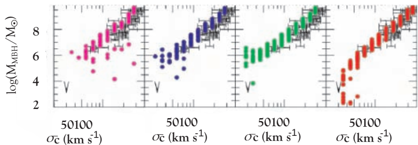
Gráficos M_{bh} - \sigma_c para cuatro modelos de formación de ANSs. Los tres primeros (magenta, azul y verde) son propuestos por Volonteri et al. (2008), y se basan en fusiones jerárquicas (en árbol) de halos de materia oscura. El cuarto (rojo) es propuesto por otros autores y considera que los ANSs se forman a partir de otros más pequeños, remanentes del colapso de estrellas de Población III. Las barras de error se toman de mediciones reales para M_{bh} y \sigma_c
