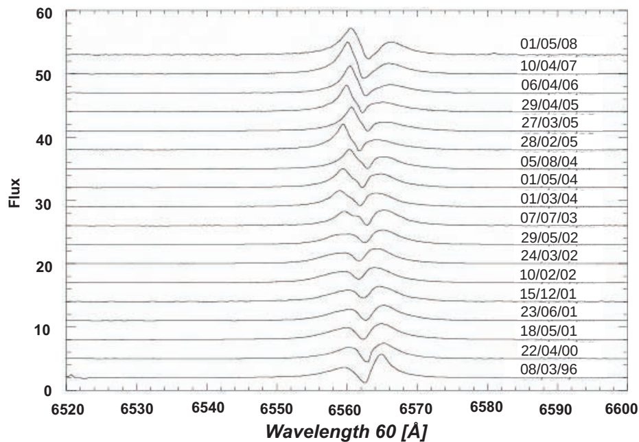
Figura 7: 48 Lib. Variaciones del perfil H durante el periodo 1996 al 2008
