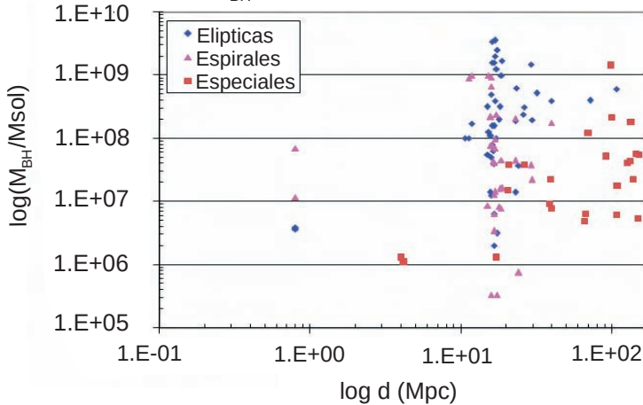
Gráfico 9: M_{BH} vrs Distancia al Centro de la Galaxia
