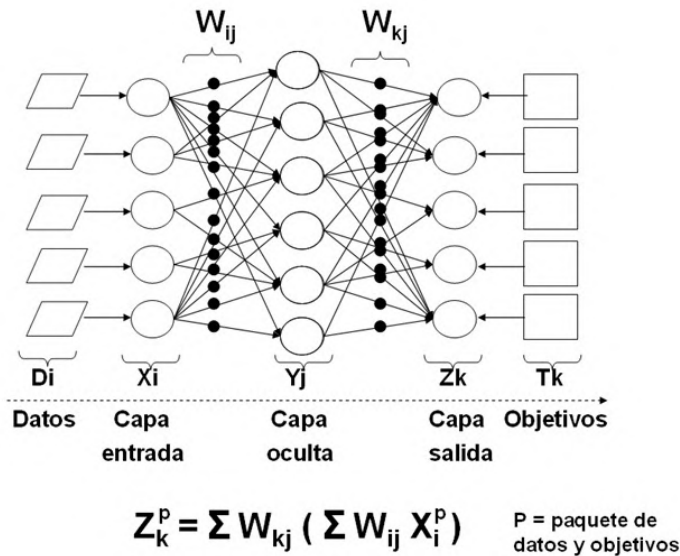
Figura 5.2 Representación de los niveles una RNA.
