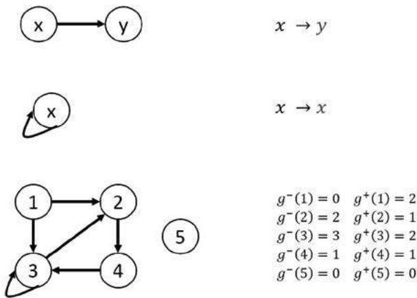
Figura 2. Grafos dirigidos
