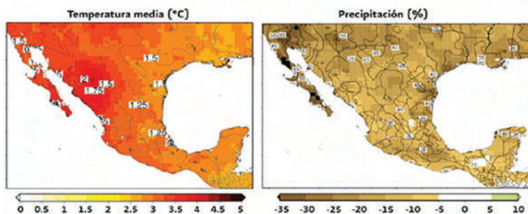
b) Escenario de emisiones A1B (medias)
