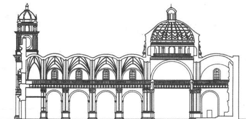
Iglesia de la Compañía de Jesús en el Cuzco, corte trasversal
