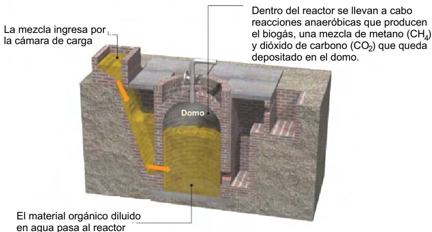
Fig.4 Biodigestor de domo fijo
