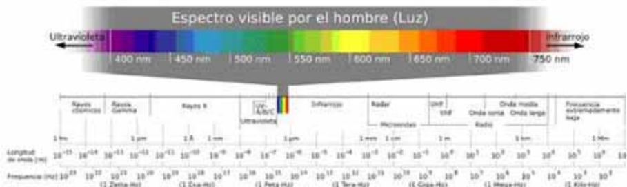
Figura 65. Espectro electromagnético
