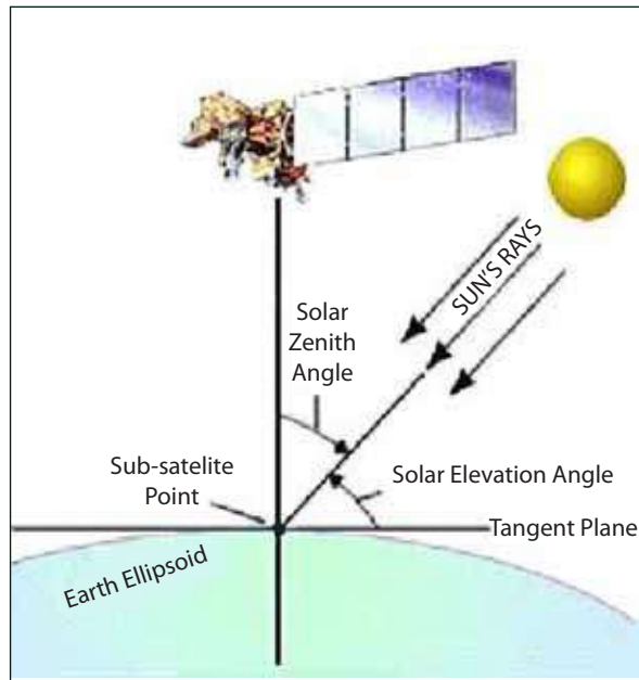
Figura 68. Ángulo de elevación solar
