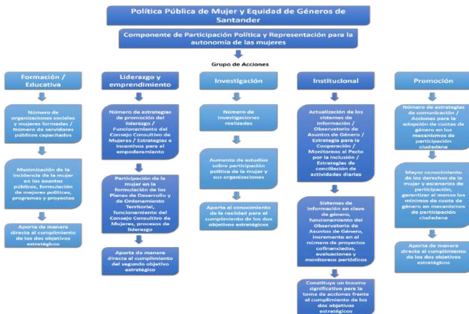
Gráfico 4. Modelo lógico.
